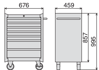
■ WS207 ローラーキャビネット寸法
