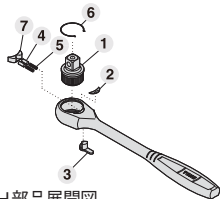
RH4H 部品展開図
